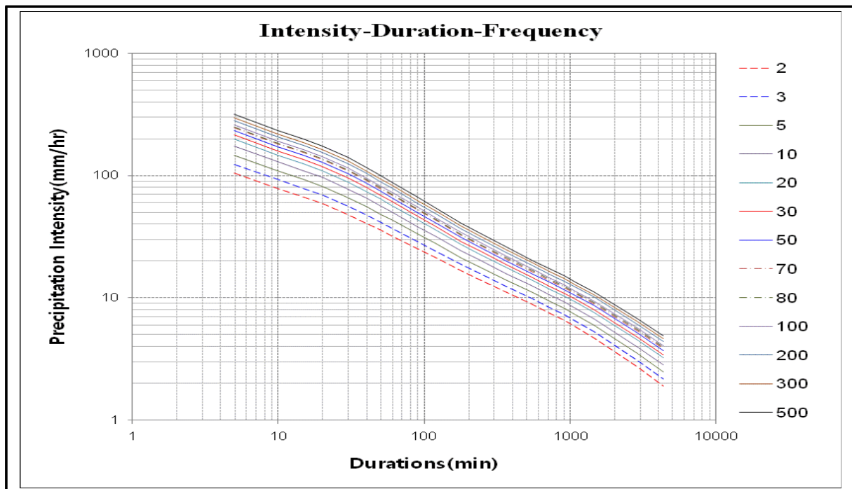
【그림 24.9】 균위지역 IDF곡선
