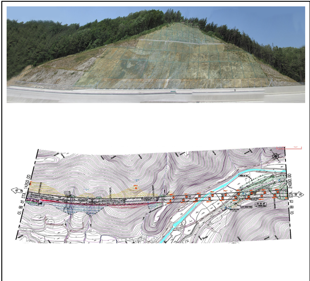
【그림 24.14】 상주절토24 검토대상 비탈면구간
