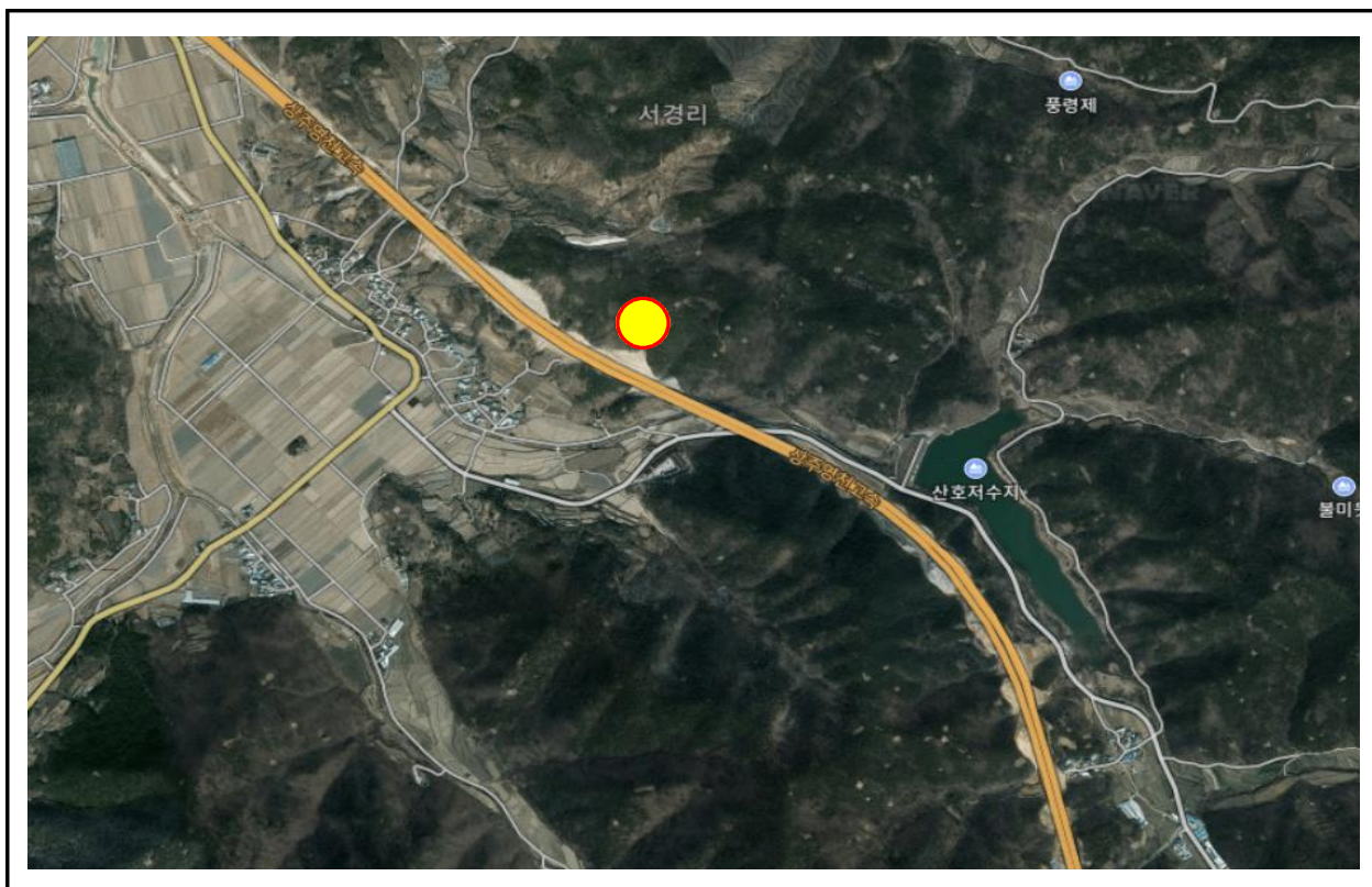
【그림 24.13】 상주절토24 검토대상 비탈면구간
