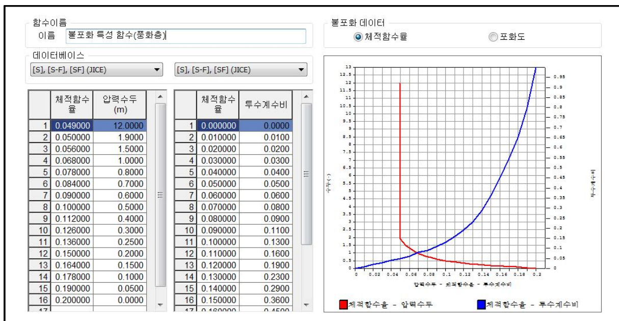
【그림 24.15】 압력수두-체적함수비(포화도)-투수계수비 함수
